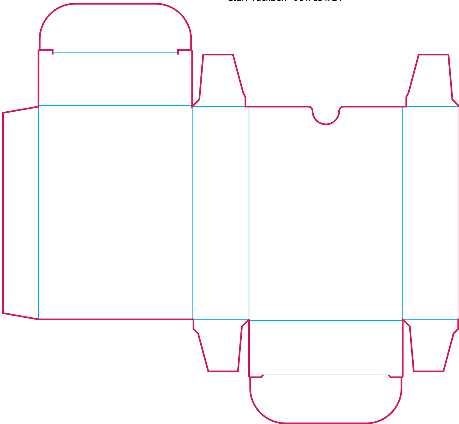
Étui / Tuckbox - 90 x 65 x 24
